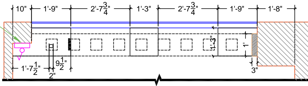
PLAN (WALL-D)
