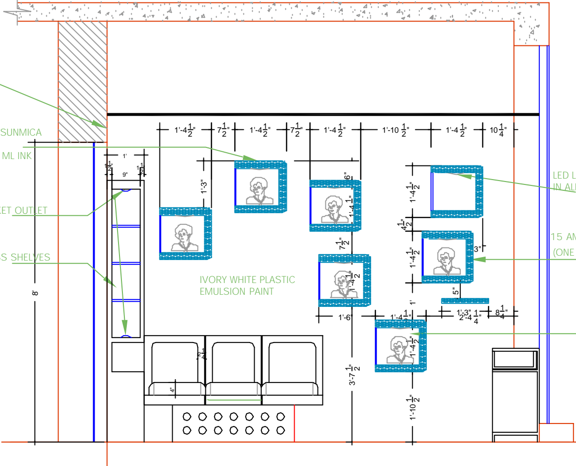
ELEVATION (WALL-C)
