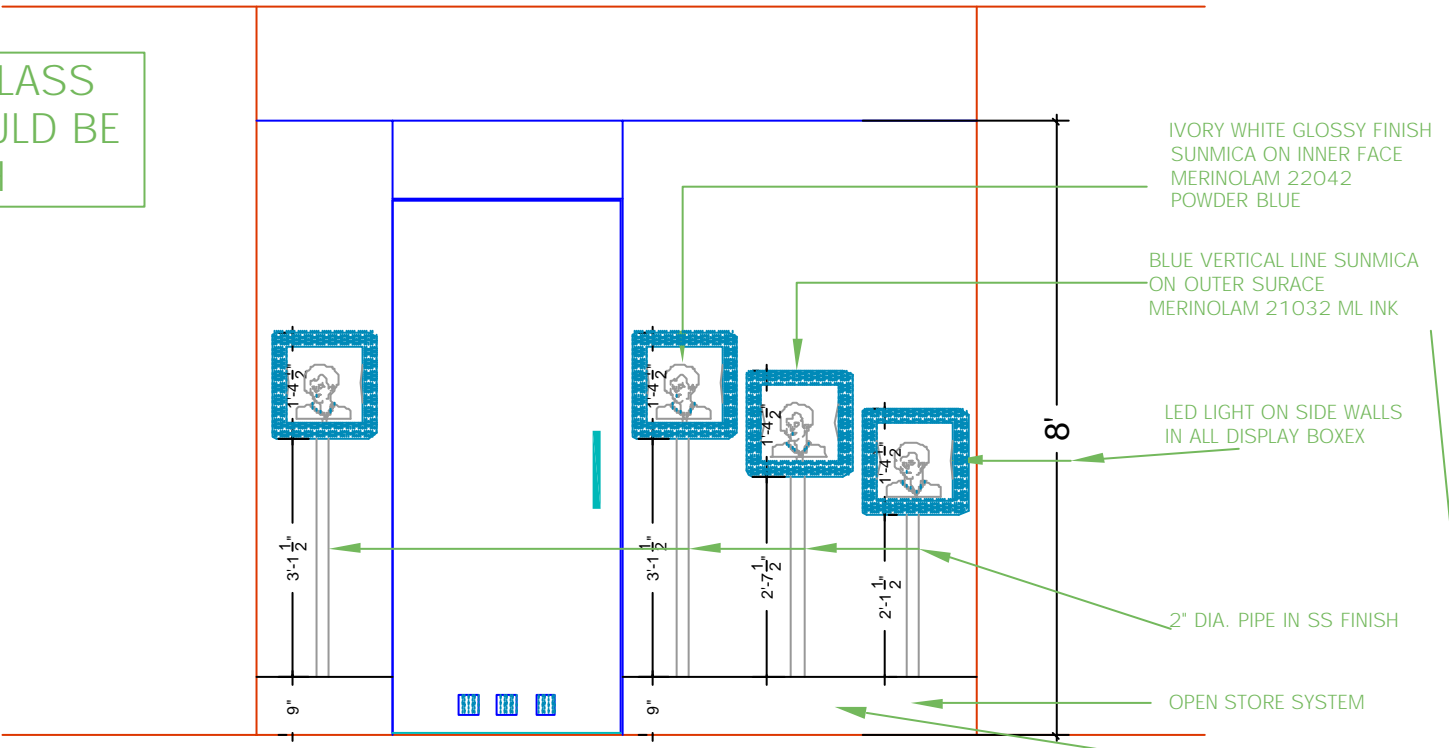
ELEVATION (WALL-B)
