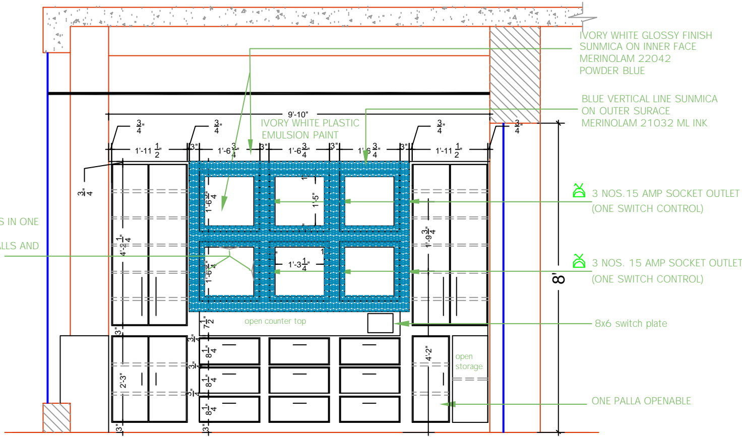
ELEVATION (WALL-A)
