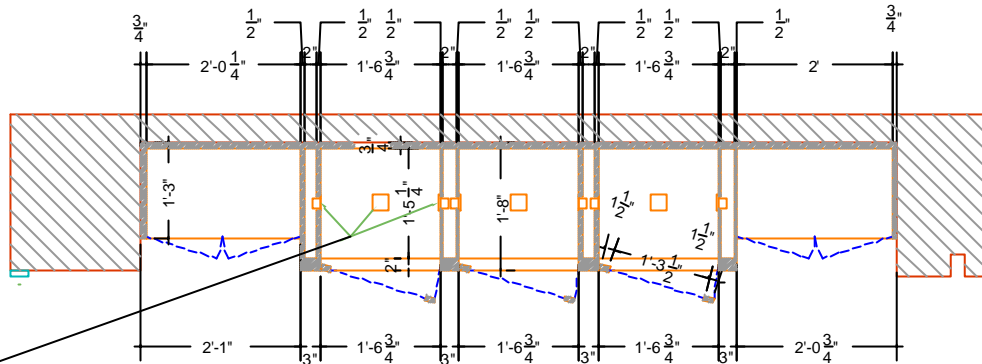
PLAN (WALL-A)
